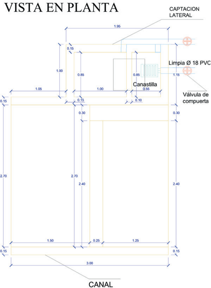
Figura 3. Vista en plata de la captación y la cámara de sedimentación
